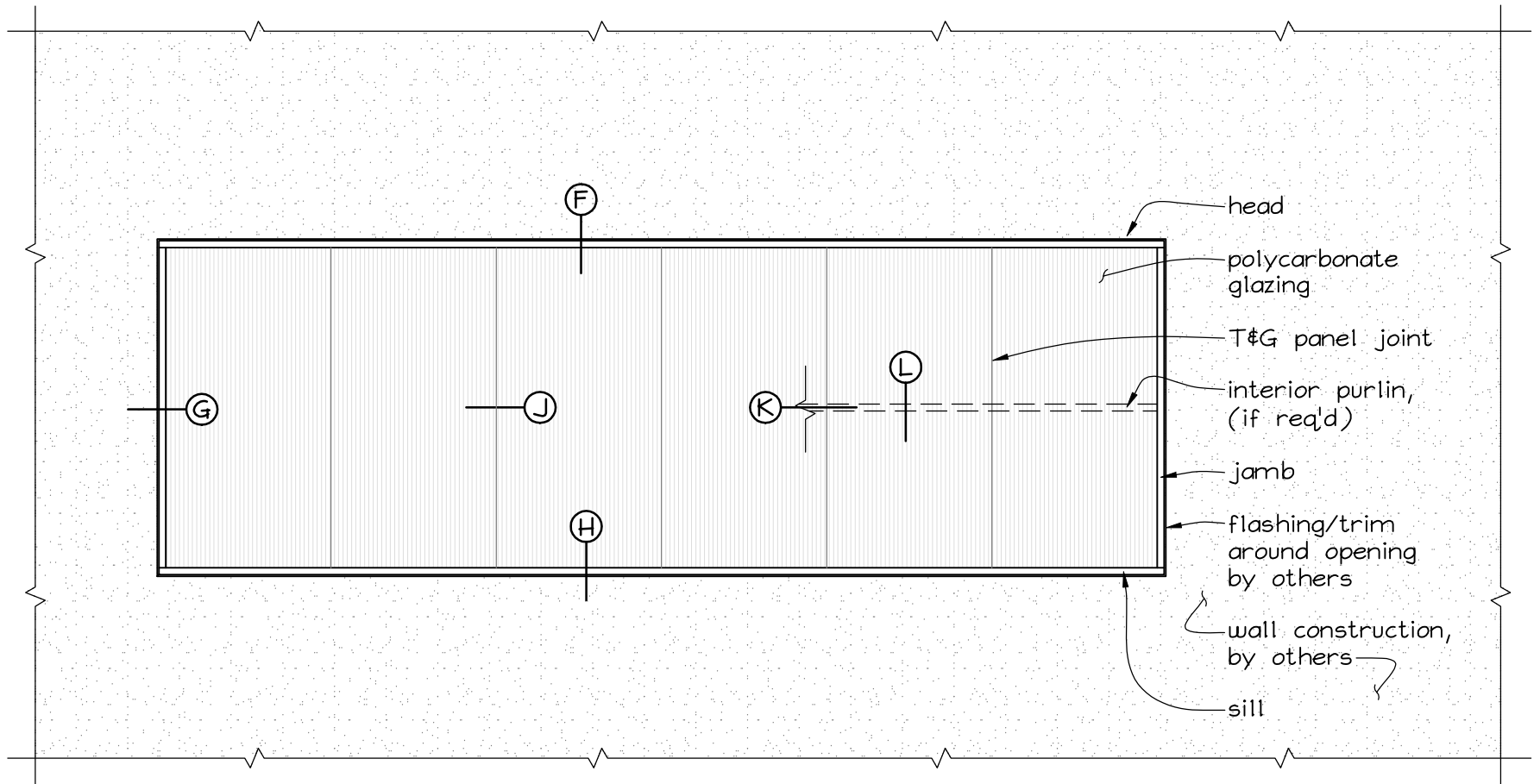
Modular System Scale: \frac{1}{4}" = 1'-0"
